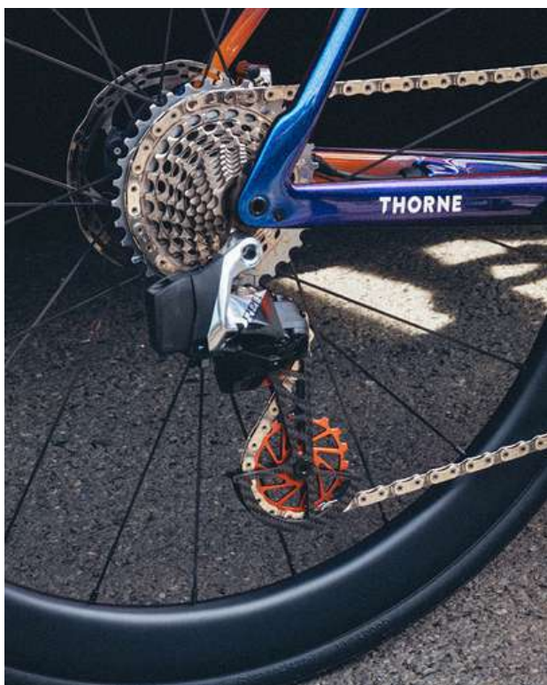
CARBON CERAMIC DERAILLEUR
